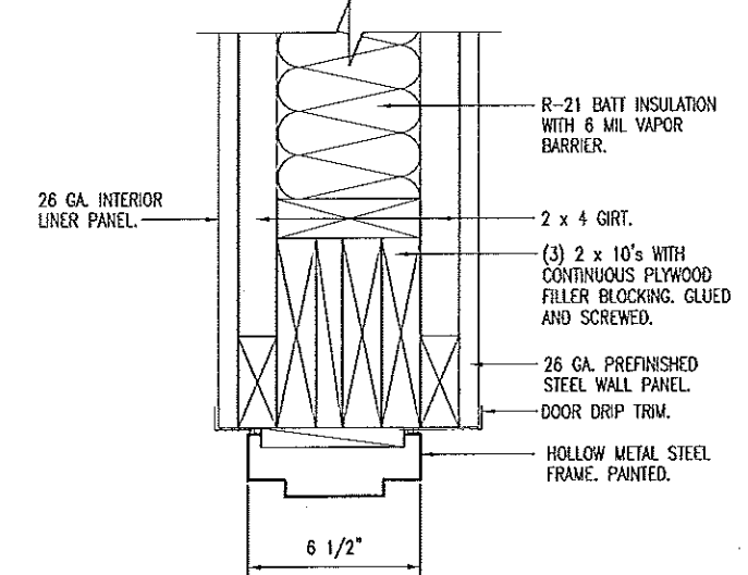
C 14 DOOR HEADER/JAMB SCALE: 1-1/2" = 1'-0"
