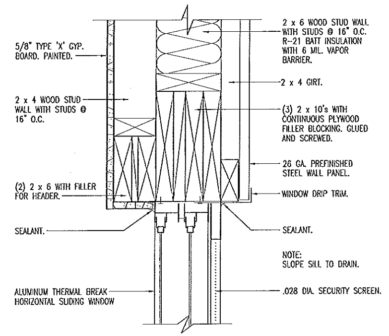
G 14 WINDOW HEAD SCALE: 1-1/2" = 1'-0"
