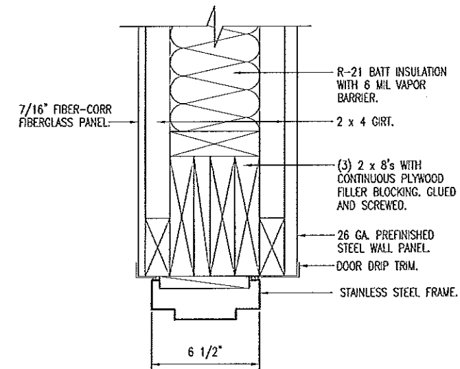
C 15 DOOR HEADER/JAMB SCALE: 1-1/2" = 1'-0"
