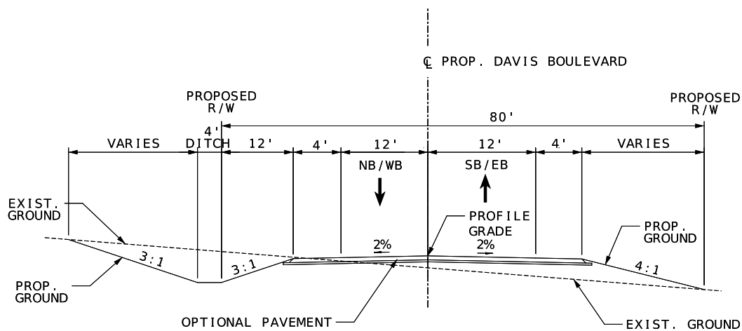
PROP. DAVIS BOULEVARD STA. 94+65.00 TO STA. 107+00.00
