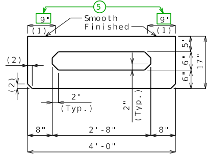
DIMENSIONS
