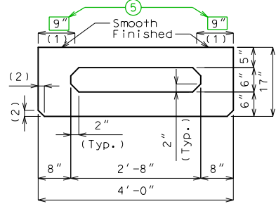
DIMENSIONS
