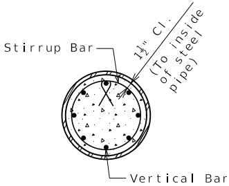
SECTION A-A 5
