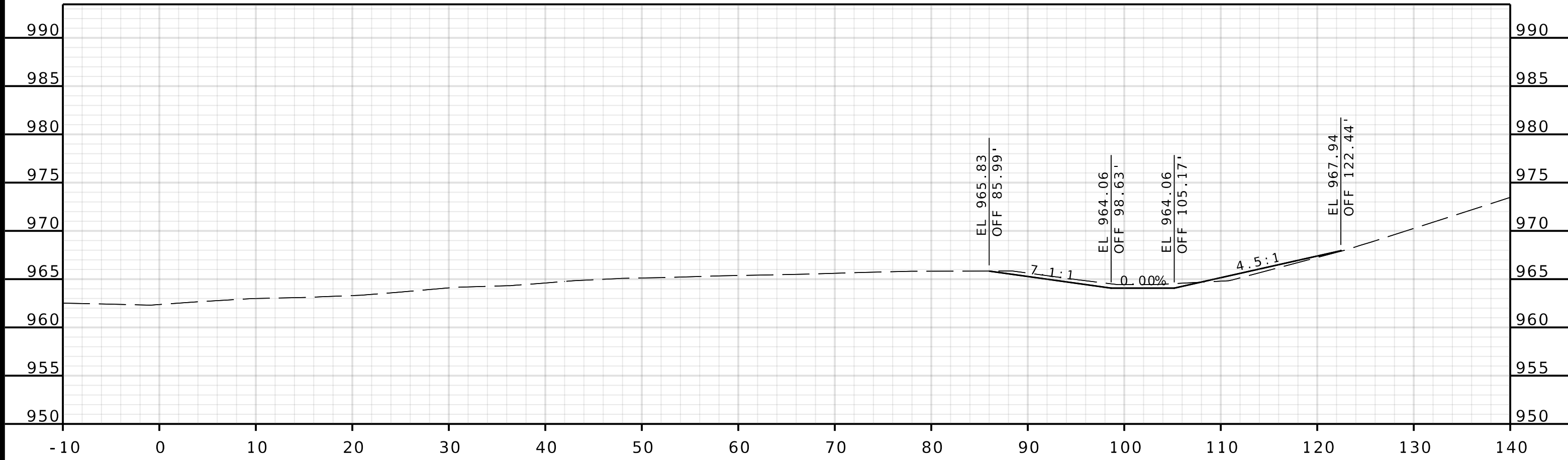
STA 943+25.00
