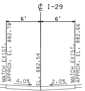
SEC. C-C 899+97.53 (I-29)
