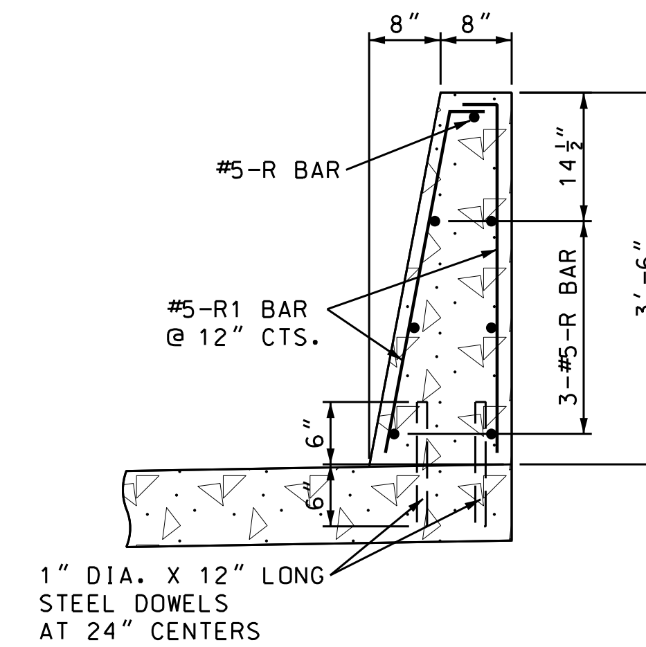
SECTION A-A
