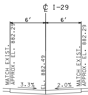
SEC. E-E 901+00.00 (I-29)
