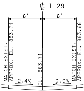
SEC. B-B 898+50 (I-29)
