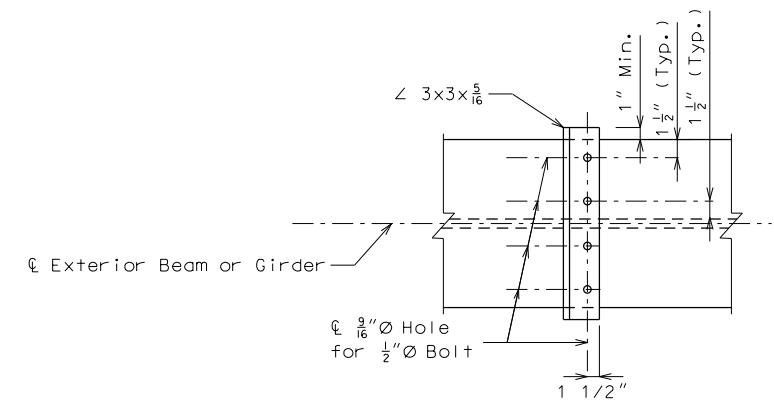
SECTION D-D
