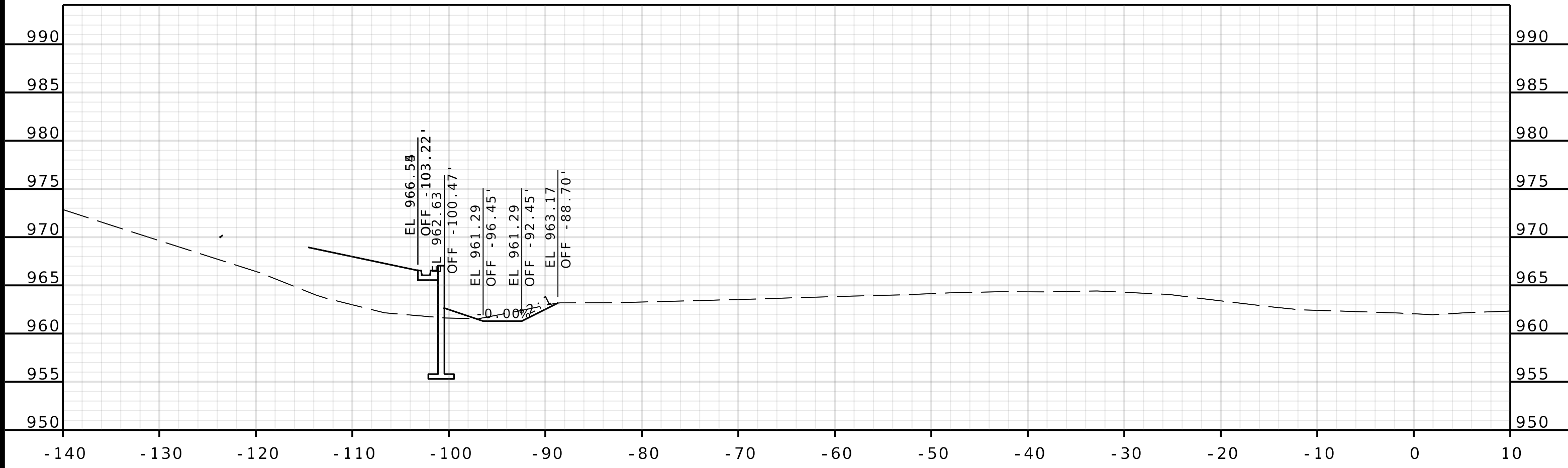
STA 942+75.00
