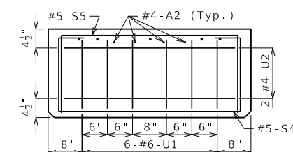
ELEVATION A-A
