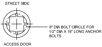
POLE DETAIL SCALE: N.T.S.
