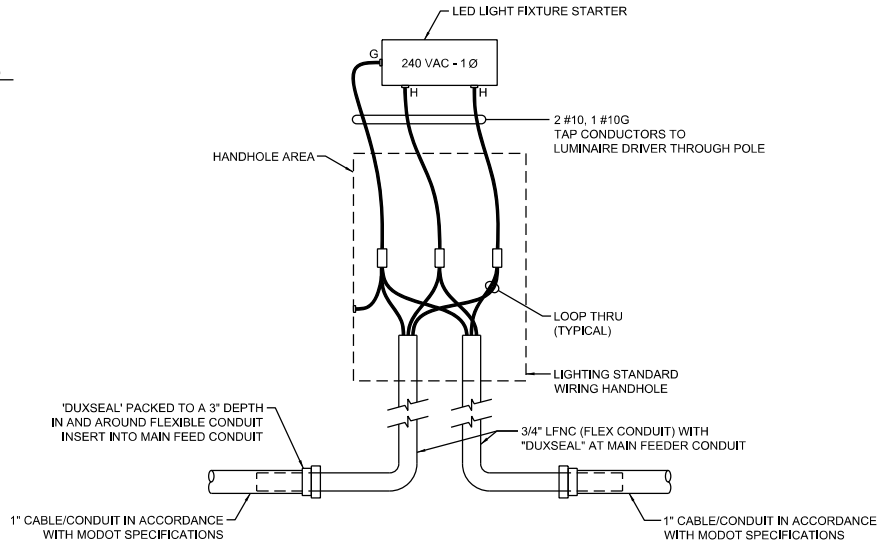
POLE DETAIL SCALE: N.T.S.
