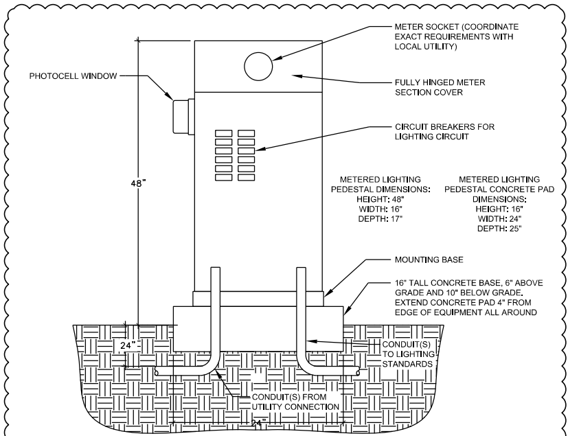
METERED LIGHTING PEDESTAL DETAIL SCALE: N.T.S.
