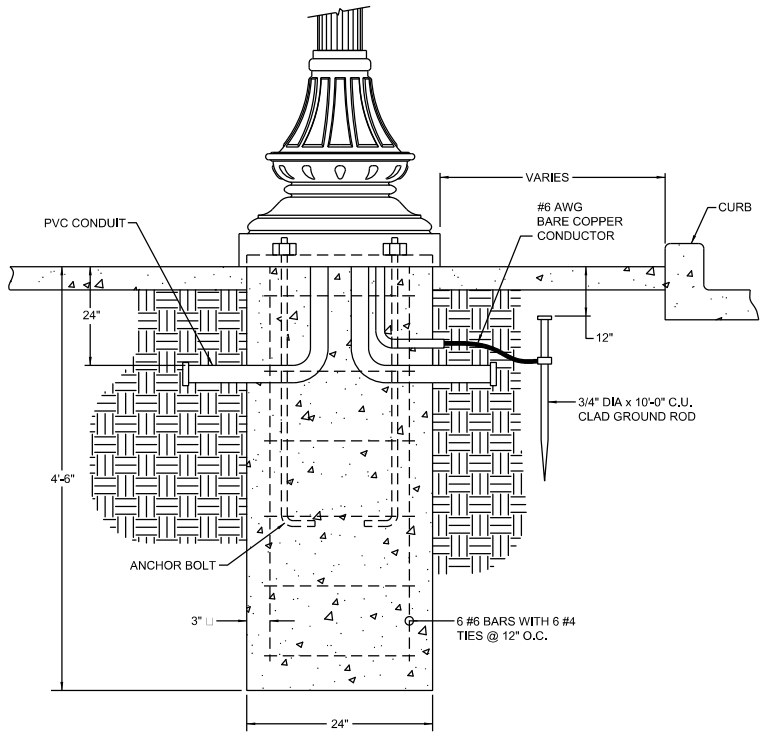
POLE BASE MOUNTING DETAIL SCALE: N.T.S.
